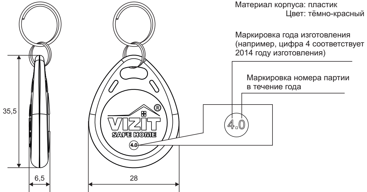
Рисунок 1 - Ключ VIZIT-RF3.1
