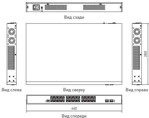
Рис. 1 — Габаритные размеры TSX-U-2GX/SFP-24GTP-R
