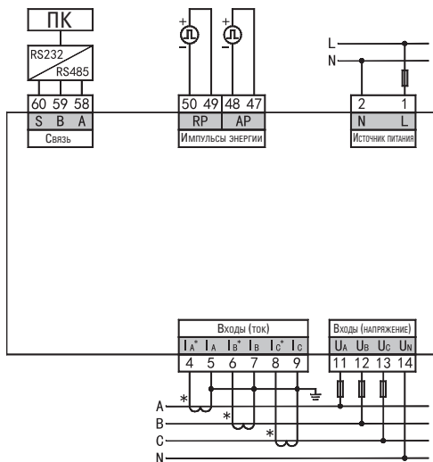
Рис. 4 Расположение клемм
