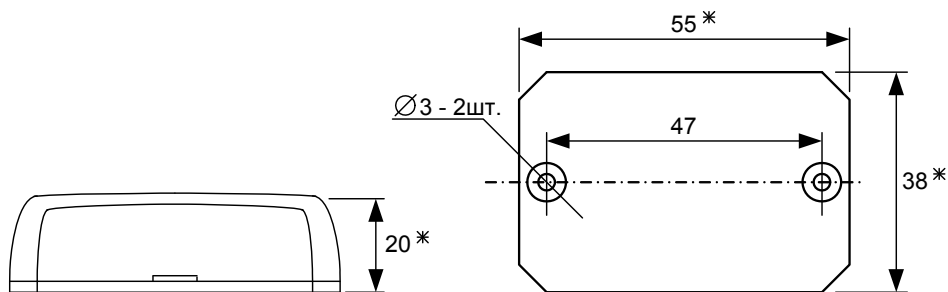
Рисунок 1 Габаритно-установочные размеры
