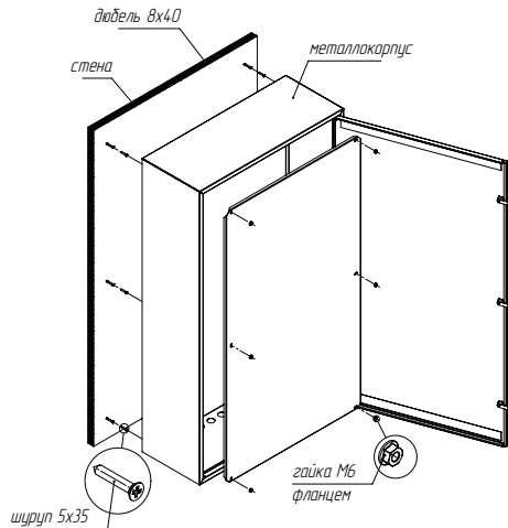
Рис. 1. Схема монтажа
