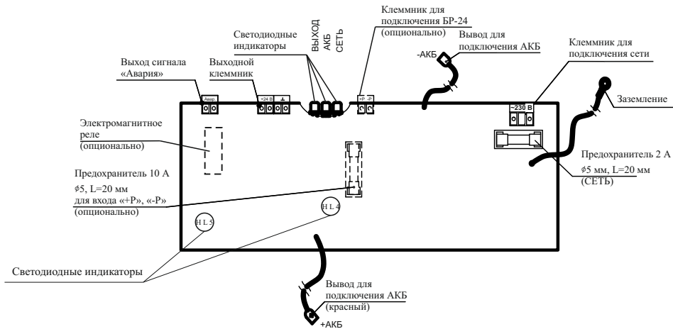
Рисунок 1 – Плата источника
