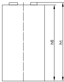
Рисунок 1 – Габаритные размеры LR03, LR06, LR14, LR20
