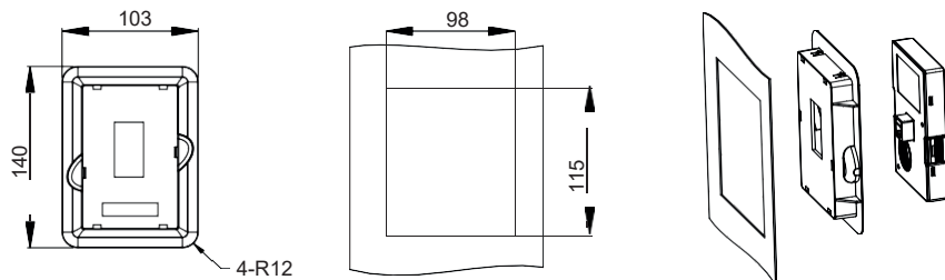
Установочные размеры
