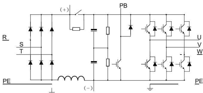
Рис 3.2 Схема силовой цепи 380В (018G/022P–037G/045P)
