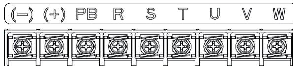
Рис 4.10 Клеммы силовых цепей ПЧ D30N4 – D37N4
