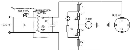
Рисунок 3 – схема фильтра
