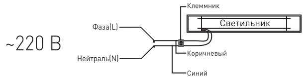
Рис.1. 220В шамчыракты токто туташтыруу схемасы
